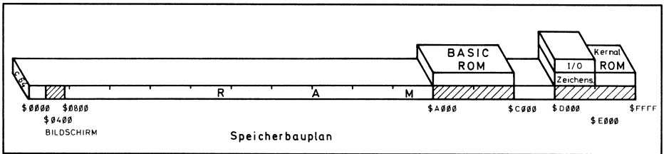
Bild 1: C64-Speicher im Aufbau
